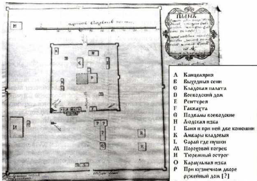
План крепости г. Якутска. Составлен А. Турчаниновым в 1768 г. Фонд НА РС(Я)
