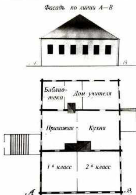
Фасад и план Якутского уездного училища. 1808 г. Фонд НА РС(Я)
