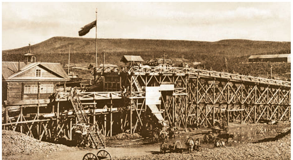
Золотопромывочное сооружение Вознесенского прииска. Конец XIX в.
