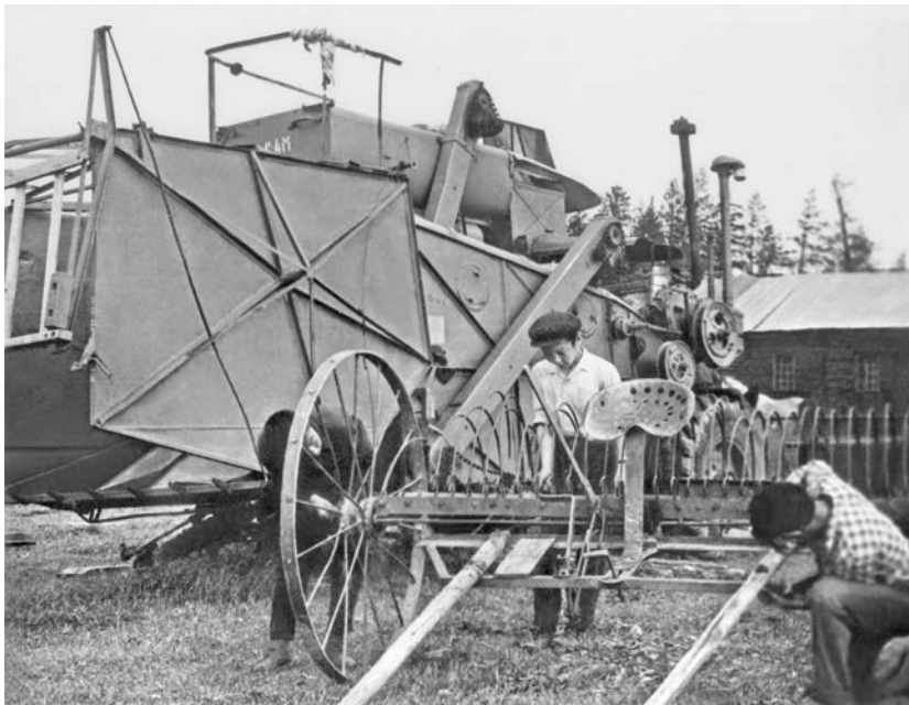
Ремонт сенокосилки. Рабочие Н.Г. Прибылых, В.И. Михайлов. 1966 г. ЯГОМИКНС, № 21899-1.
